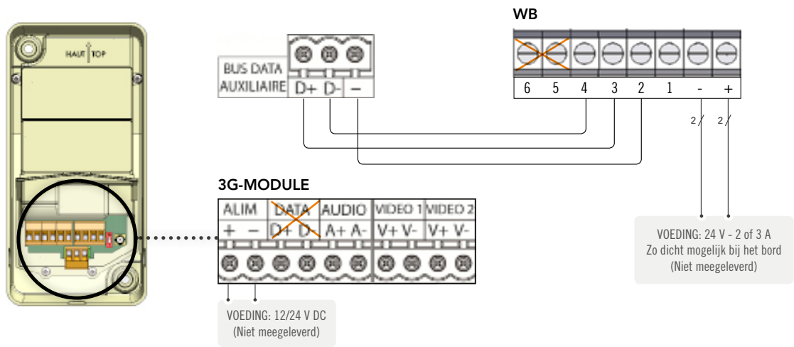
Schema 1: vereenvoudigde bedrading
